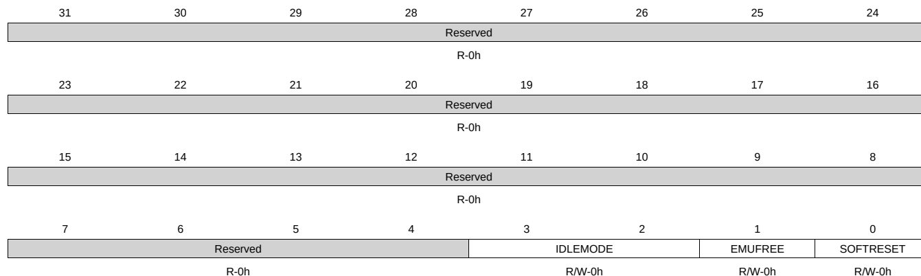
Figure 20-10. TIOCP_CFG Register
