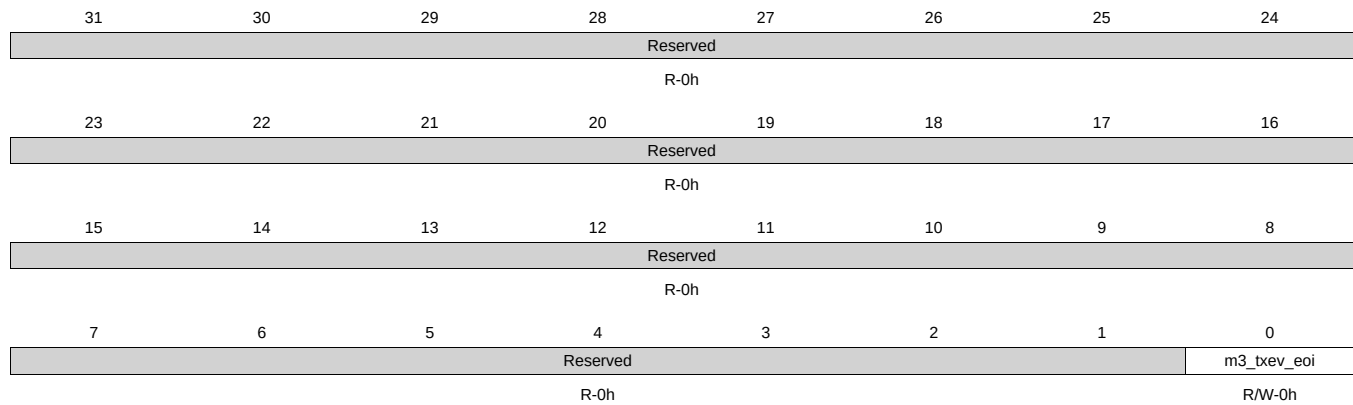
Figure 9-82. m3_txev_eoi Register
