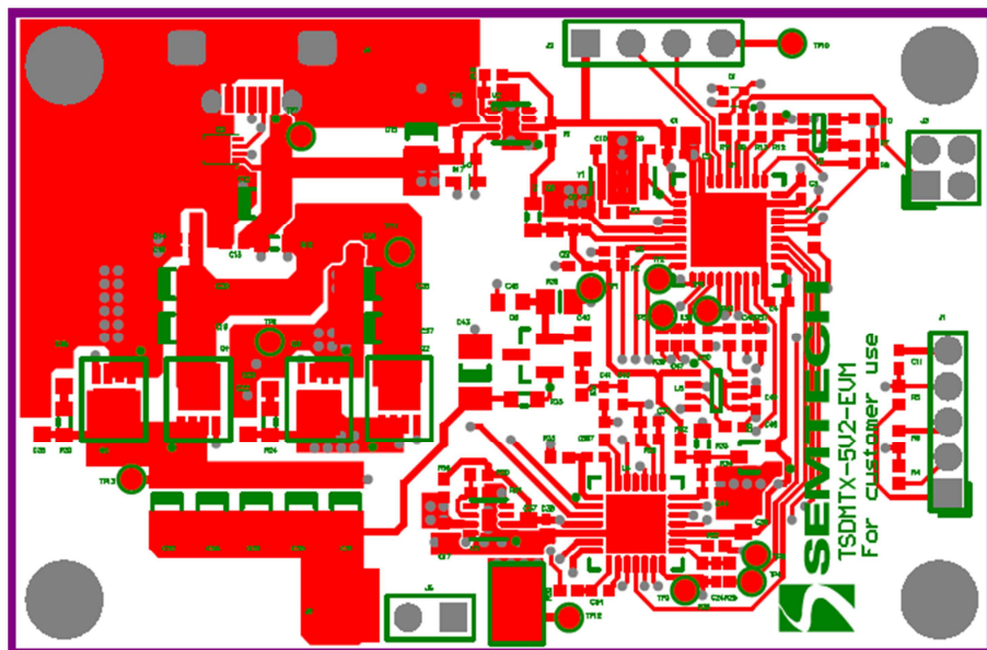
Top Layer
