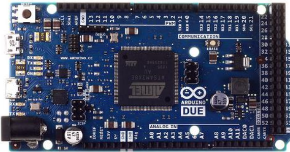
Arduino Due Front
