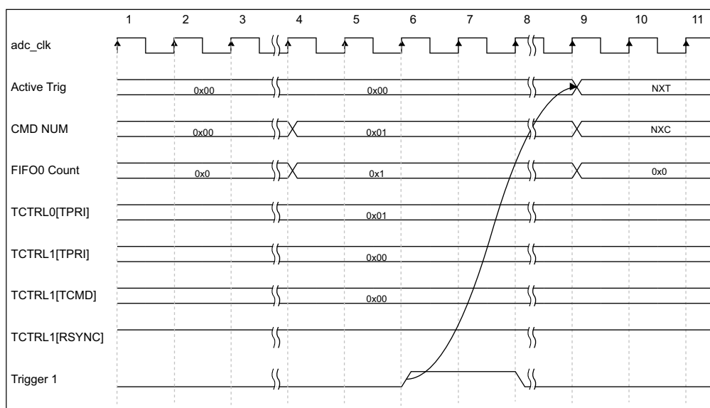
Fig 148. ADC resync example
