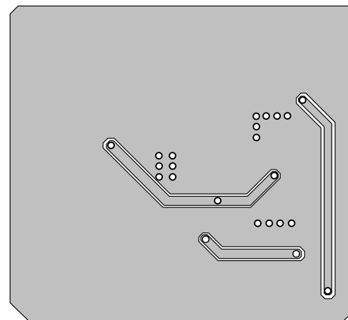
Bottom Layer
