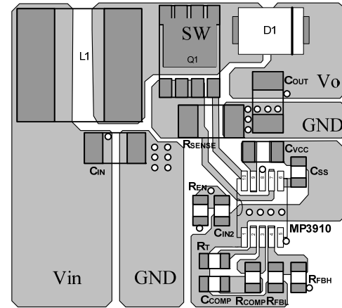
Top Layer
