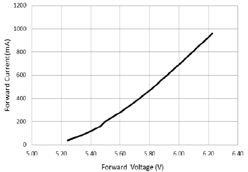
V_f ----- I_f
