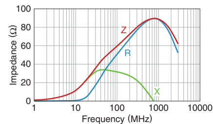
MPZ1005S600C
