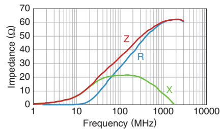
MPZ0603S330C
