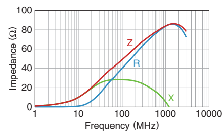
MPZ0603S470C
