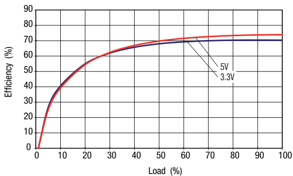
MEJ2S03XXSC
