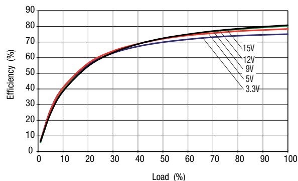
MEJ2D12XXSC
