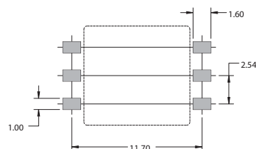
6 Pin SM
