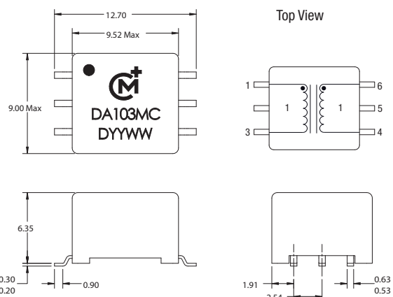
6 Pin SM
