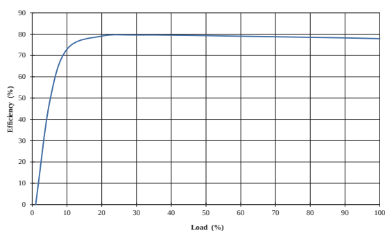
MGJ6D24XXXWMC
