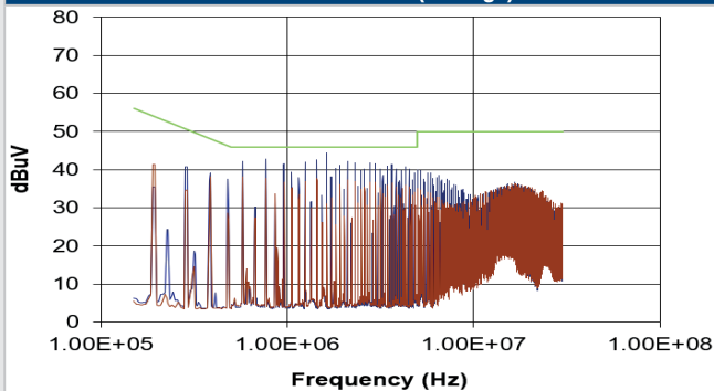
MGJ2D151509MPC (Average)
