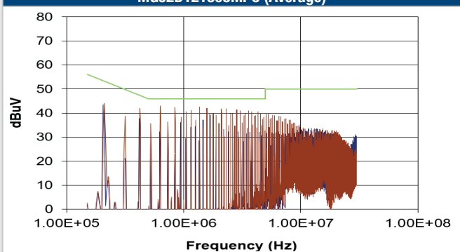
MGJ2D121509MPC (Average)
