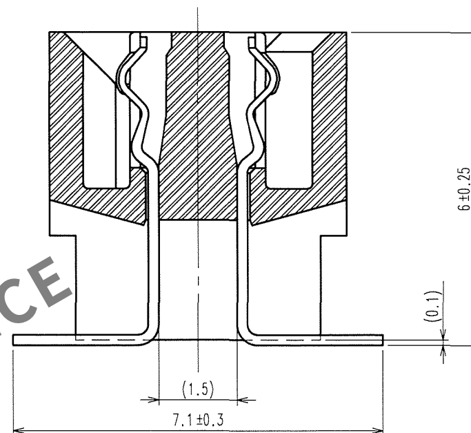
A-A (10:1)
