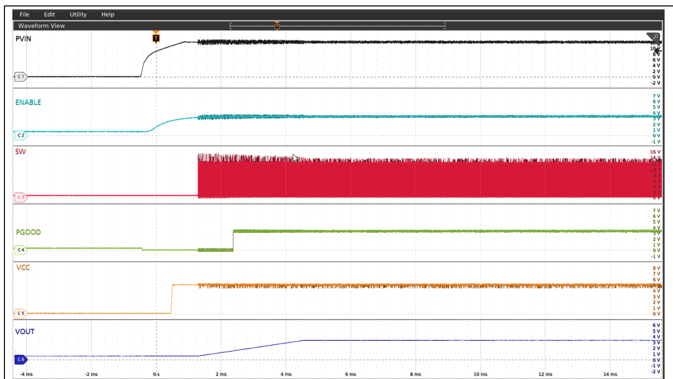
Figure 25 Start-up at 0 A load (Ch 1 : P VIN , Ch 2 : enable, Ch 3 : switch node, Ch 4 : P GOOD , Ch 5 : V DRV , Ch 6 : V OUT )
