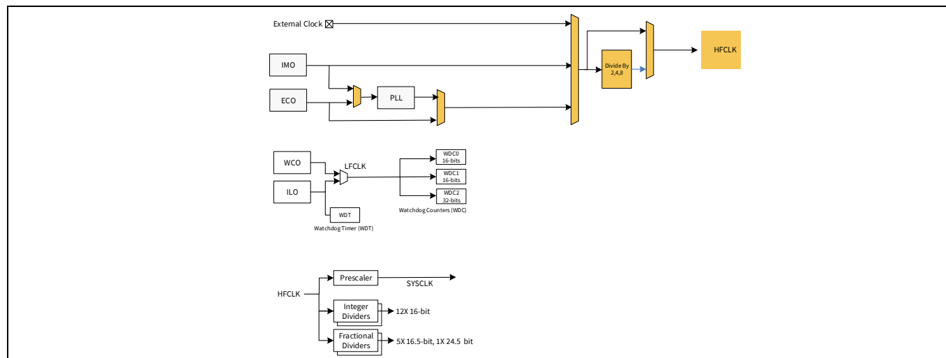
Figure 3 PSOC™ 4100S Plus MCU クロック アーキテクチャ
