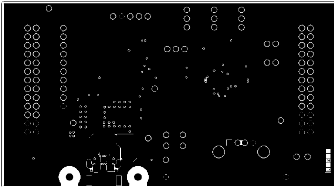
600-60412-01 REV06 GROUND1 LAYER
