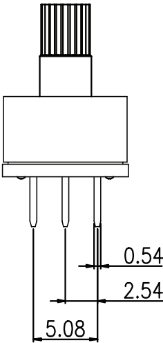
ACTUATOR
