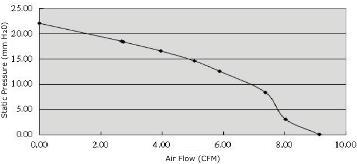
CBM-6025B-250-373
