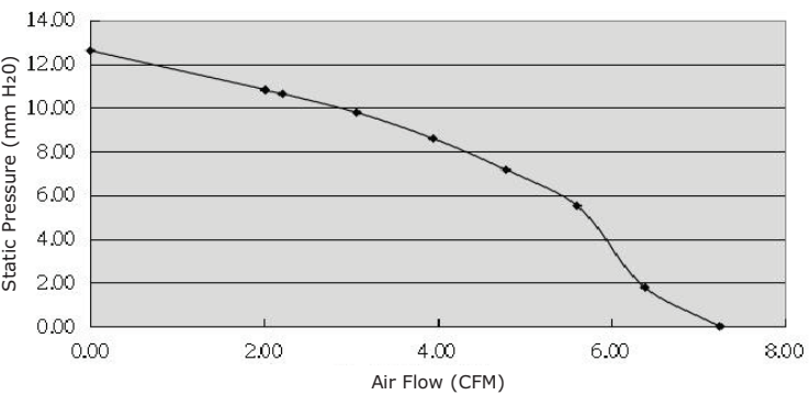
CBM-6025B-240-310
