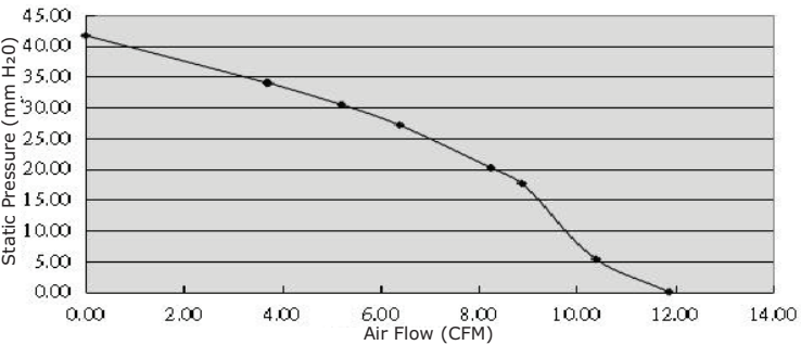
CBM-6025B-265-447
