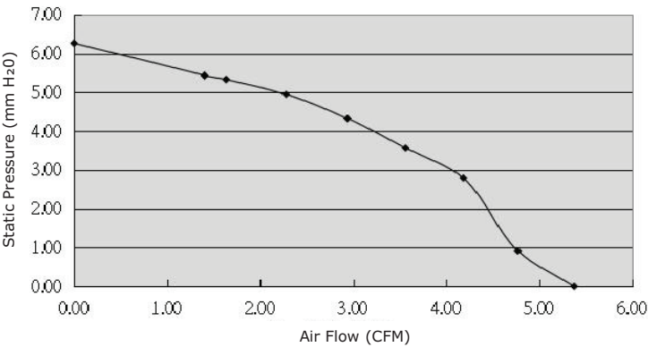
CBM-6025B-230-236
