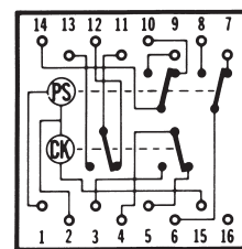
TERMINAL WIRING
