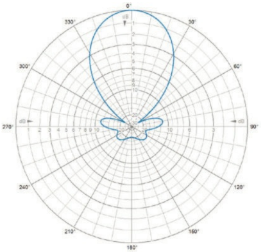
H-Plane | 445 MHz
