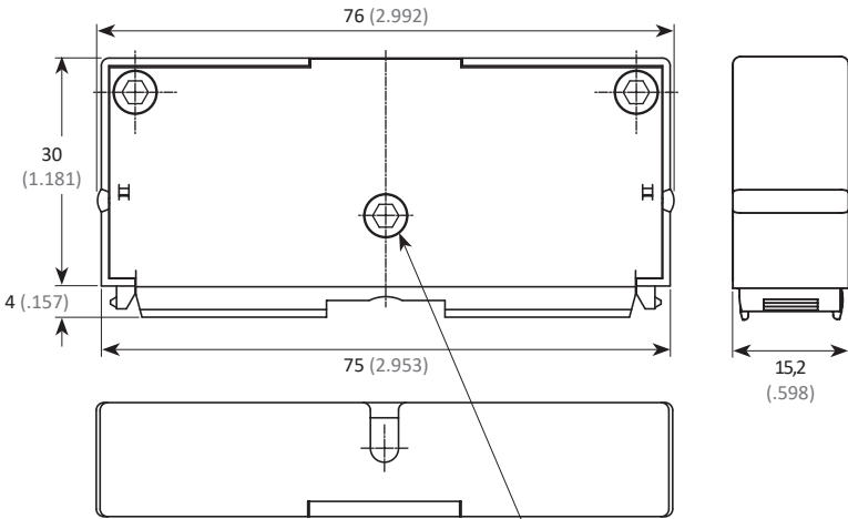
Couple de serrage de 0,5 à 0,7 N.m max. Tightening torque 0,5 N.m to 0,7 N.m maxi.
