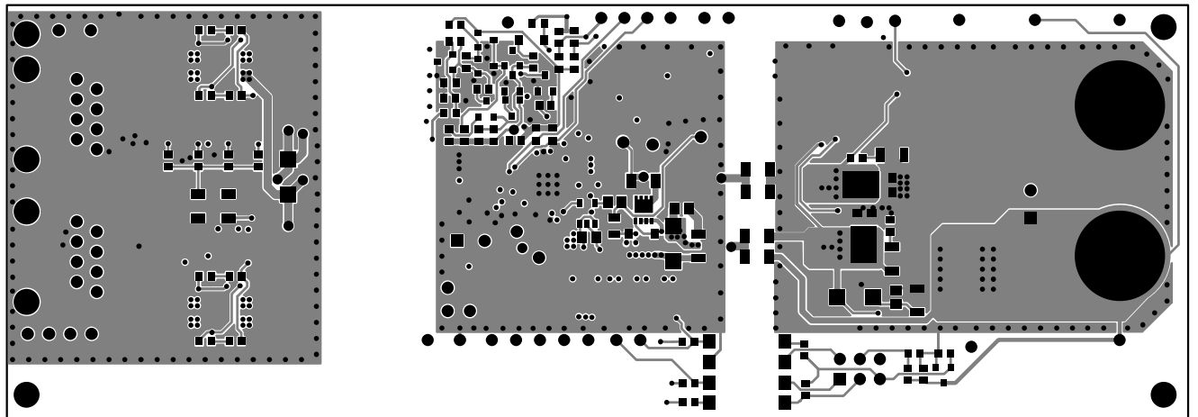
Figure 34. Bottom Layer
