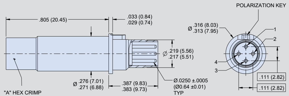
Pin Contact 854-047
