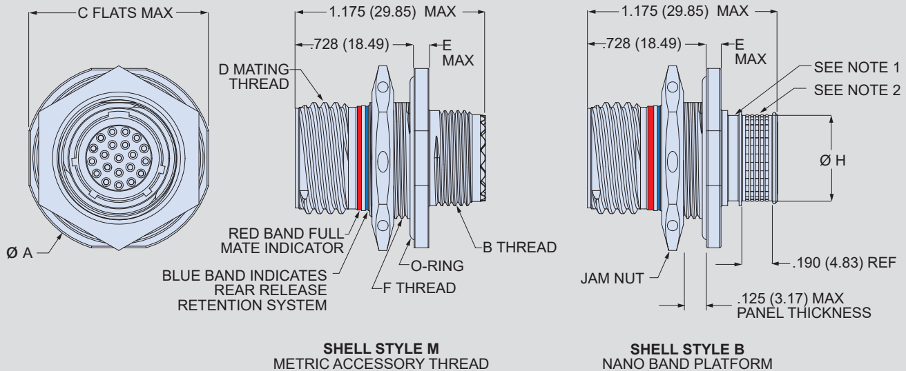
806-053 Receptacle Dimensions
