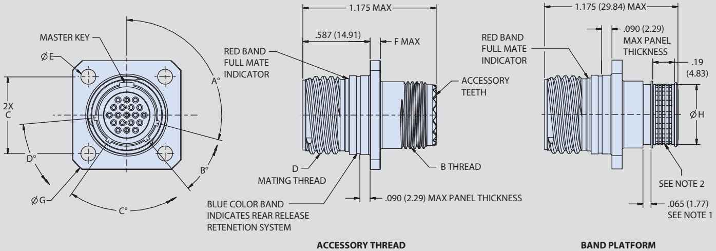
806-052 Receptacle Dimensions
