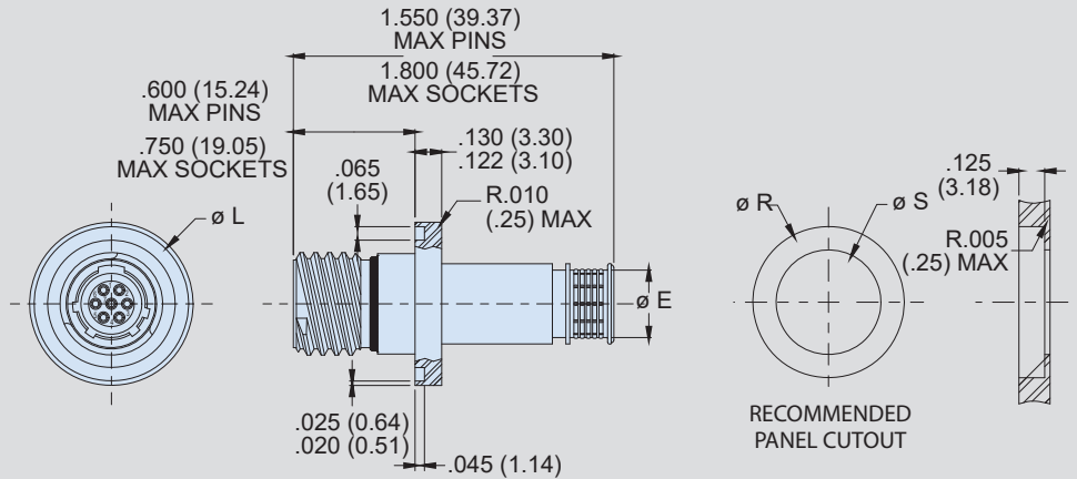
806-087-13 Weld Mount Receptacle Dimensions
