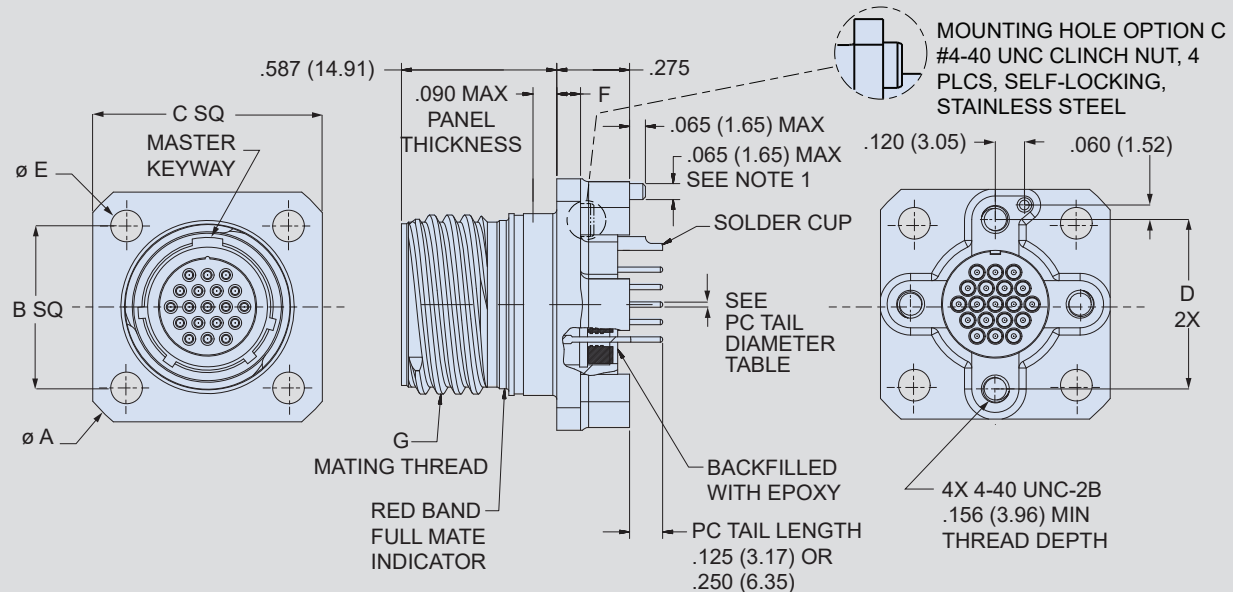
806-022 Receptacle Dimensions
