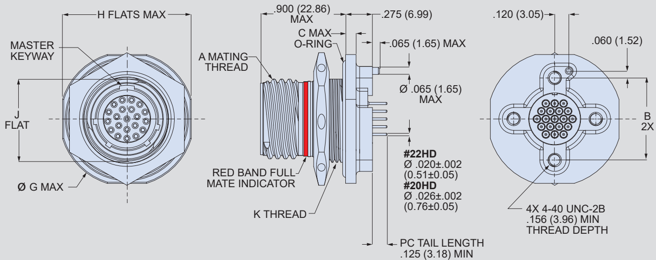
240-806-21 Receptacle Dimensions
