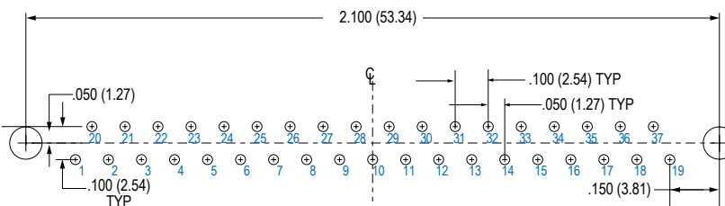
37 SOCKET
