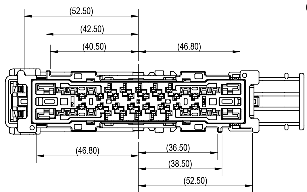
7298-7513-30 KEYWAY A
