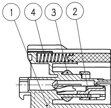
SEC. A-A
