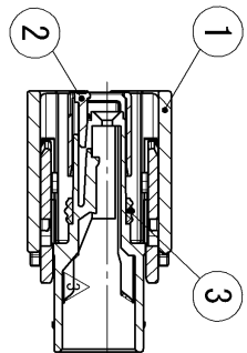
SEC. A-A
