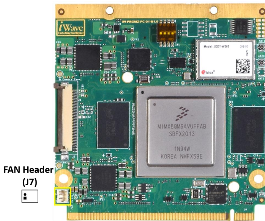
Figure 10: FAN Header
