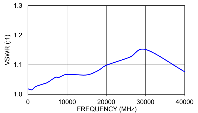
BW-KM3-2W44+ VSWR
