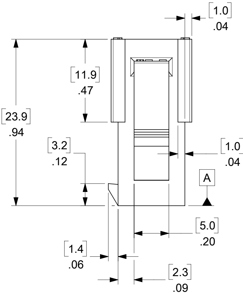
8 CKT SHOWN
