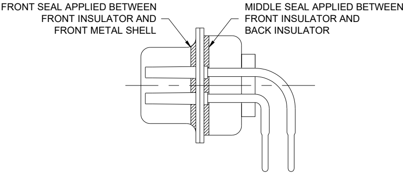
DETAIL A-A
