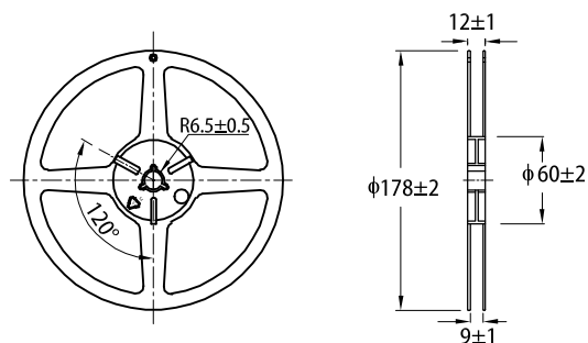
REEL DIMENSION (units : mm)
