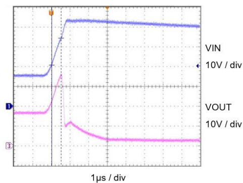
OVP Transient
