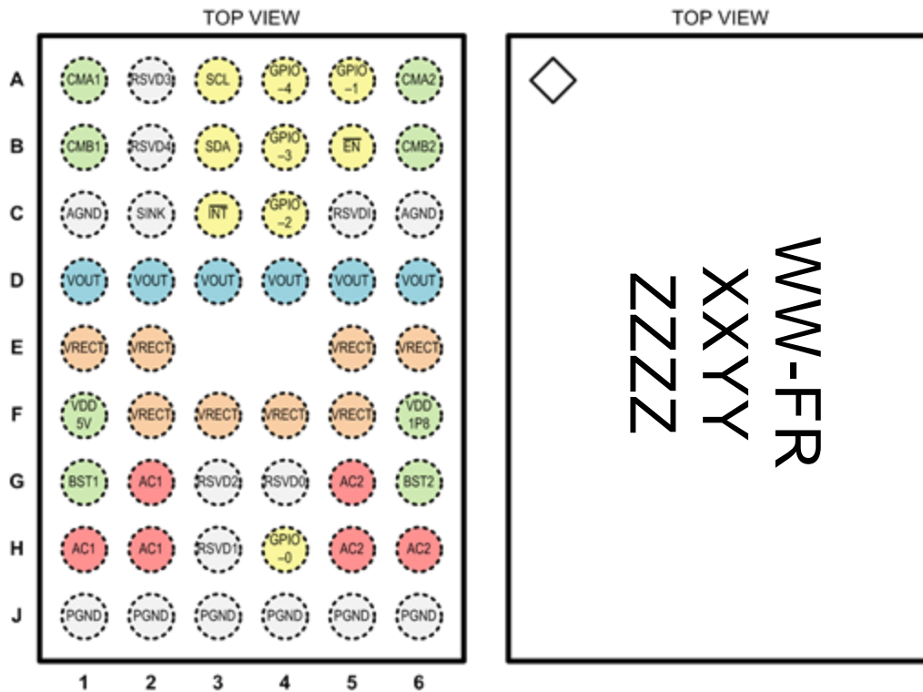
WLCSP69-52
