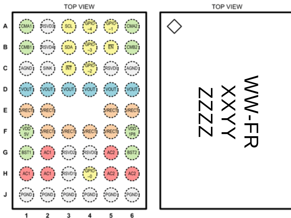
WLCSP69-52
