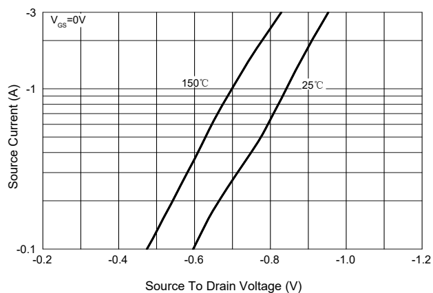
Fig.9 - I_S - V_{SD}
