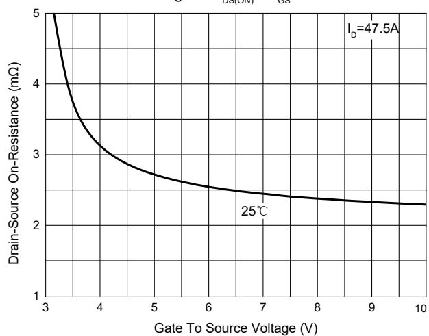
Fig. 3 - R_{DS(ON)} - V_{GS}
