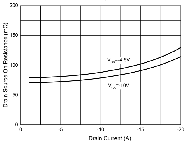
Fig. 4 - R_{DS(ON)} - I_D
