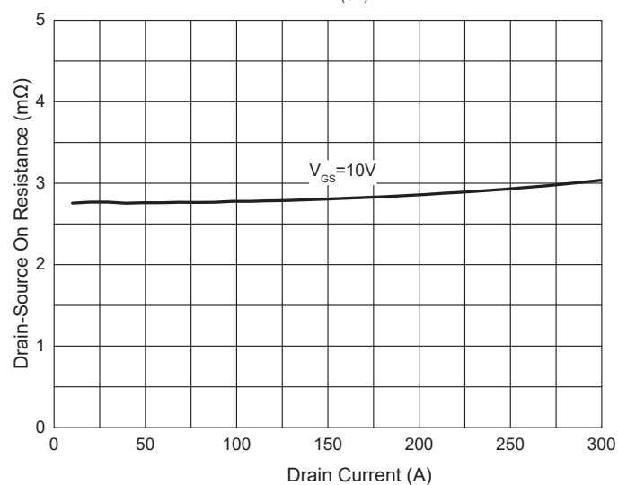
Fig. 4 - R_{DS(ON)} - I_D
