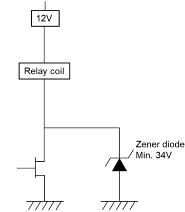
1. Using zener diode
