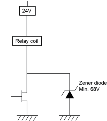
2. Using zener diode
