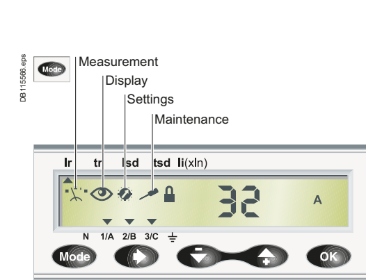
Trip unit menus
