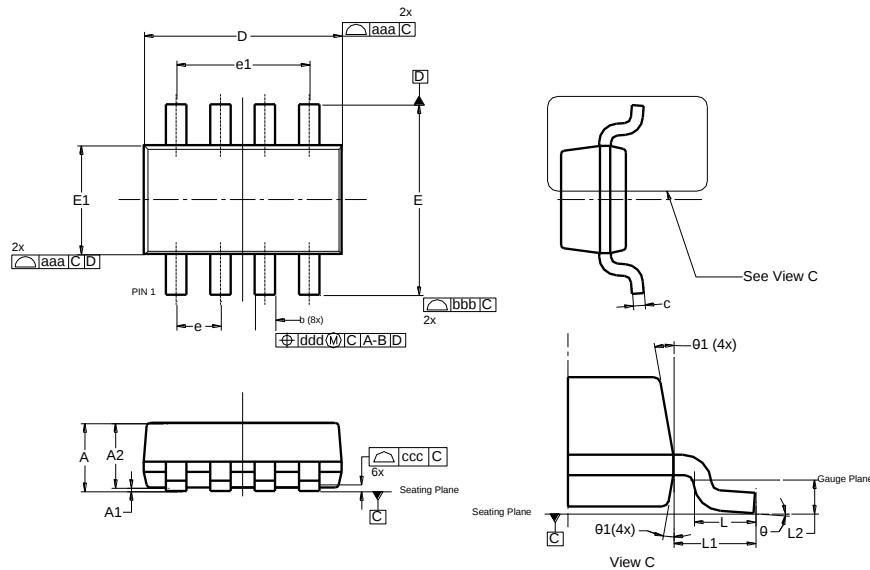
SOT28
