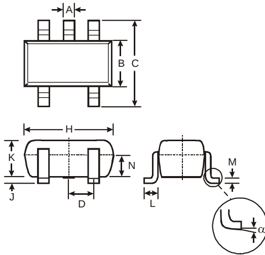
SOT25
