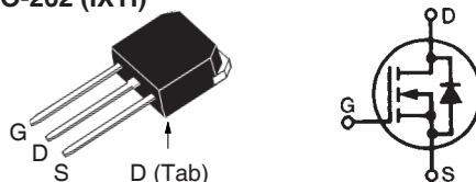
TO-262 (IXTI)
