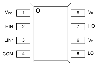
Top View: SOIC(N)-8
