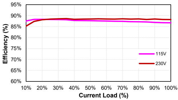
TRH50A240 (Eff Vs Io)
