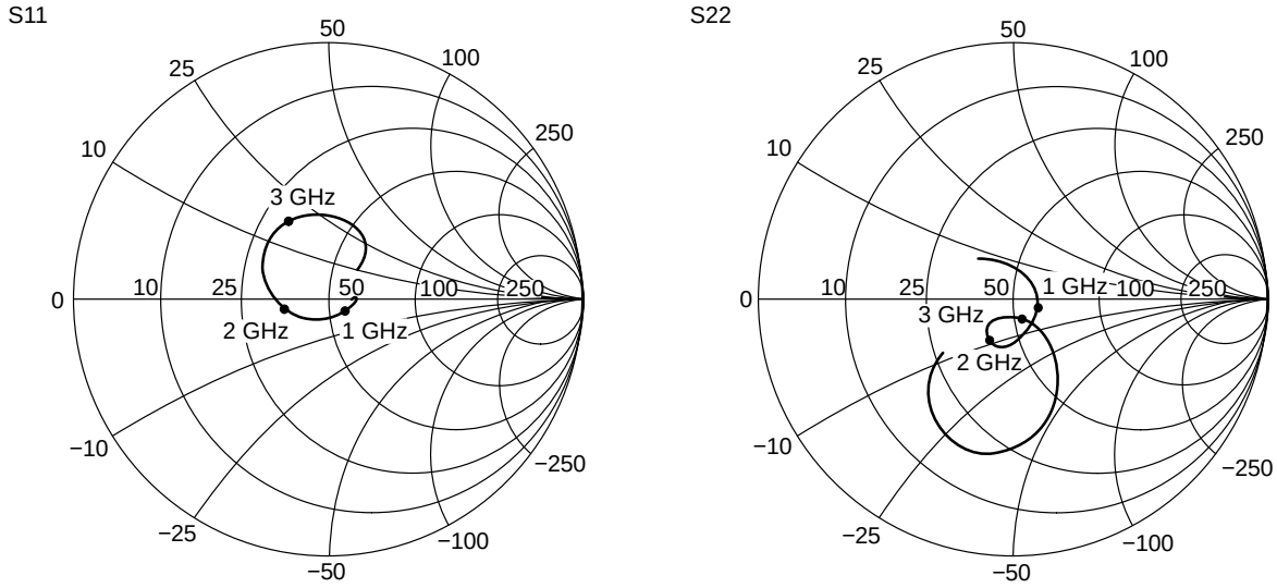
Figure 10. S Parameter
