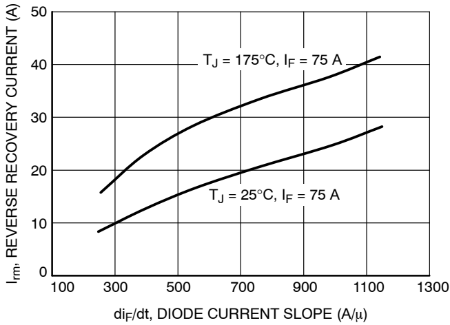
Figure 21. I_{rrm} vs. di_F/dt ( V_R = 400 V)
