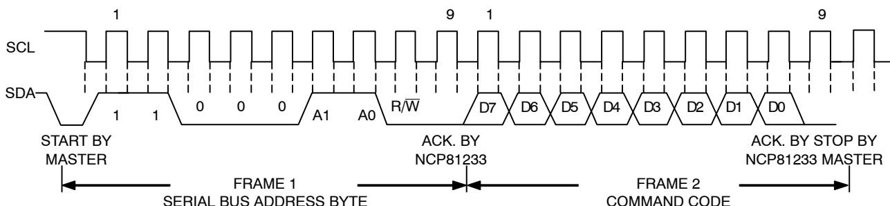
Figure 19. Send Byte
