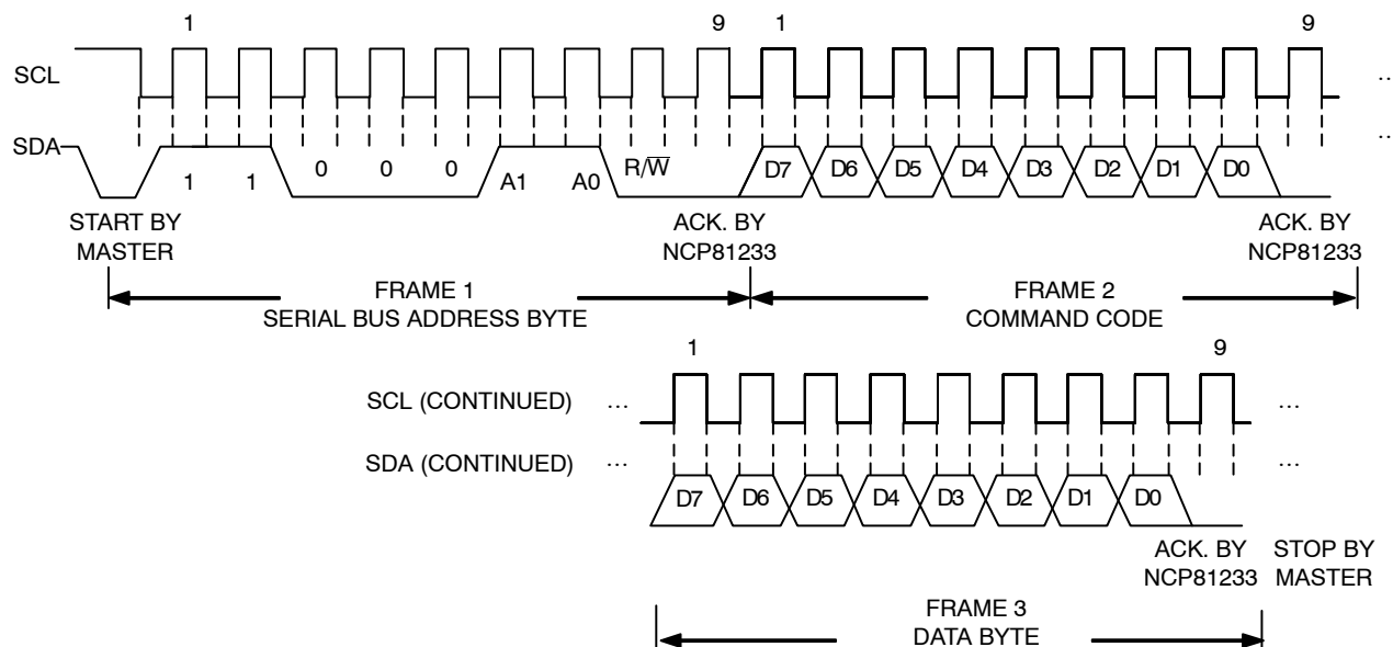
Figure 20. Write Byte
