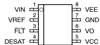
NCD5701B
