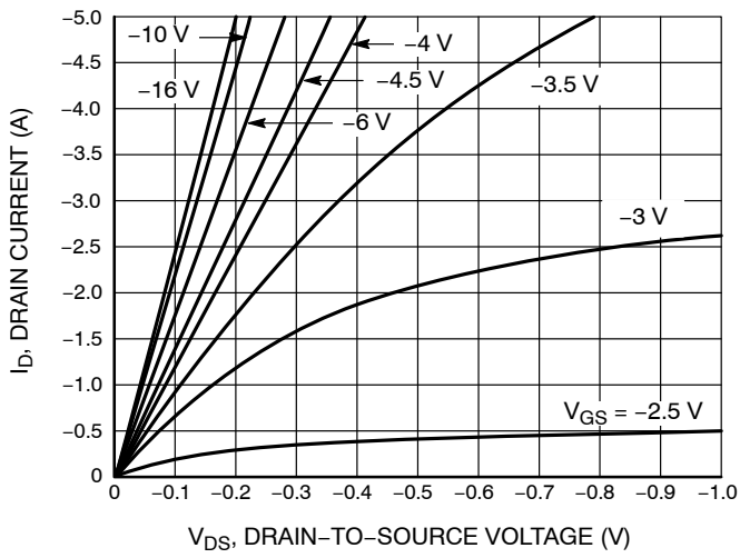
Figure 2. I_D - V_{DS}
